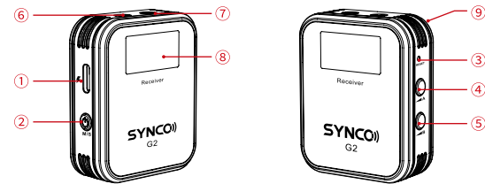
RX Ресивер
