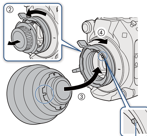
Broche d'index de l'objectif PL
